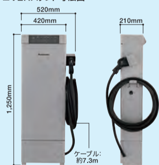
■V2Hスタンド寸法図
